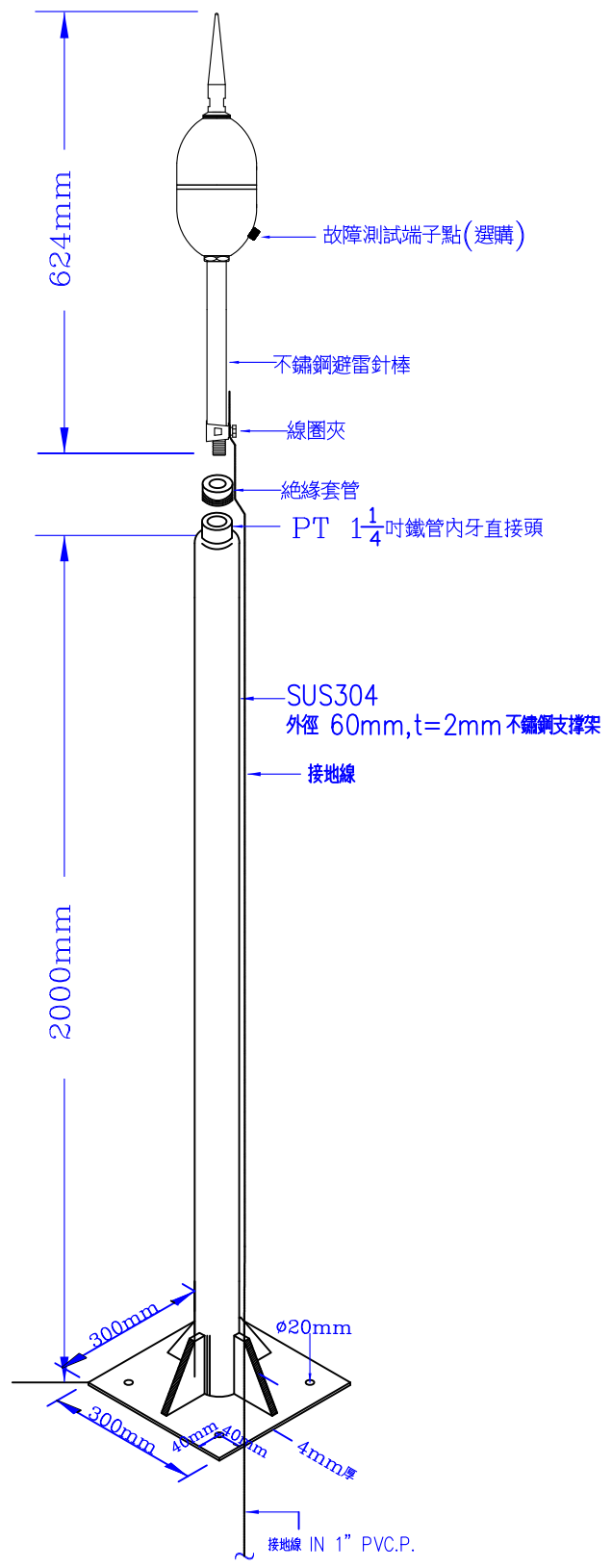
避雷針組合示意圖
